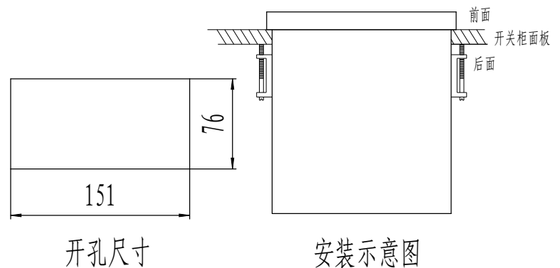
图2 安装尺寸
