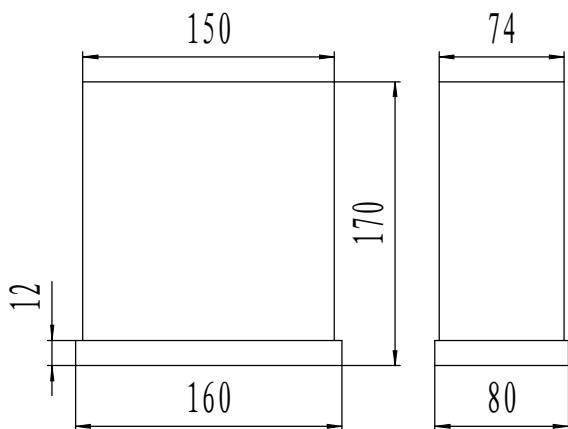
图1 外形尺寸
